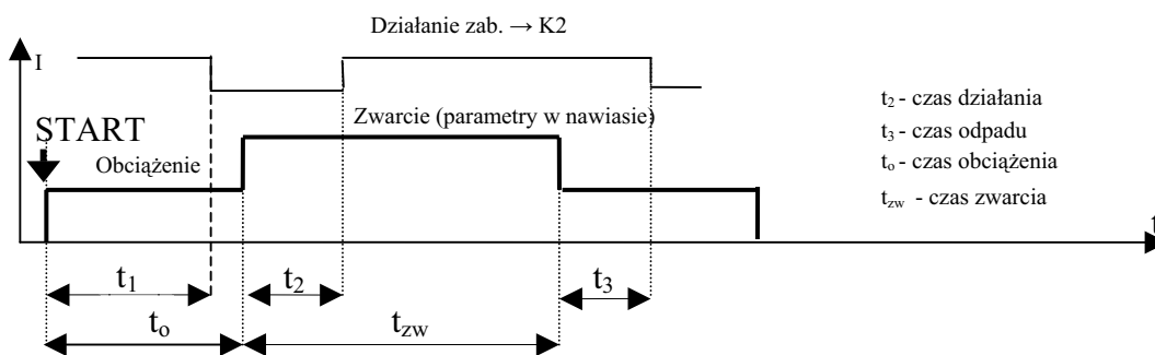
Rys. 1. Działanie urządzenia UTC-GT, tryb pracy ZWARCIE.
